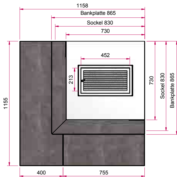
Изображение сверху М 1:20
