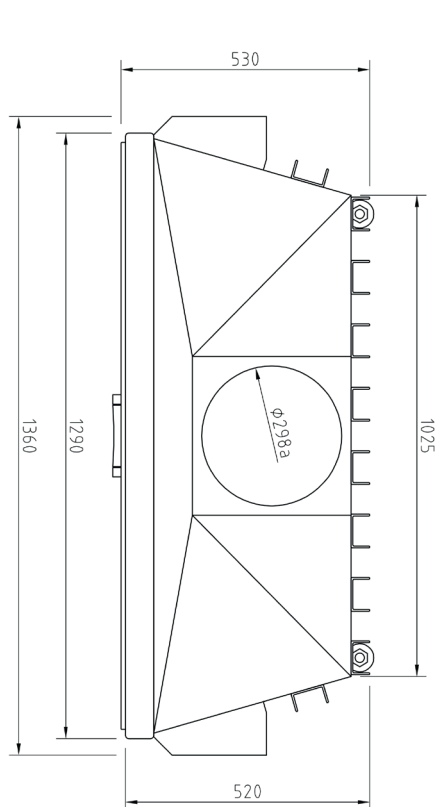
Изображение сверху М 1:10
