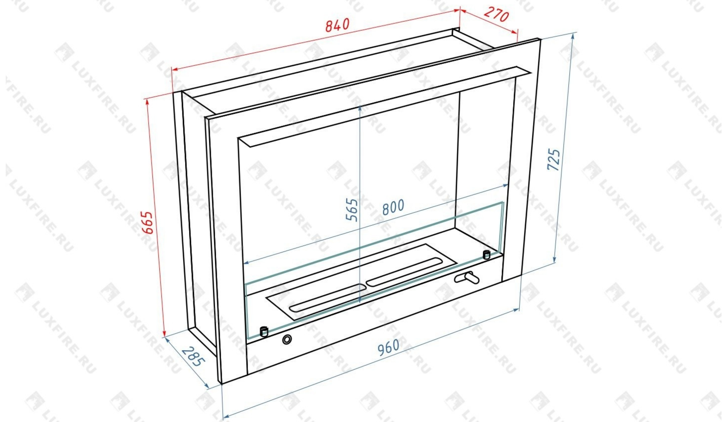
Схема Фаер Бокс 3 - 33
