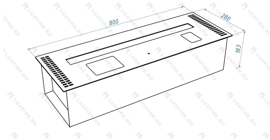
Ниша для АБК-800
